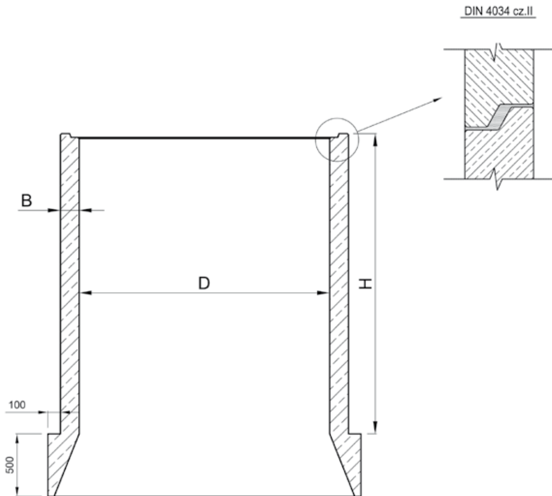
KRĄG Z NOŻEM ŻELBETOWYM
